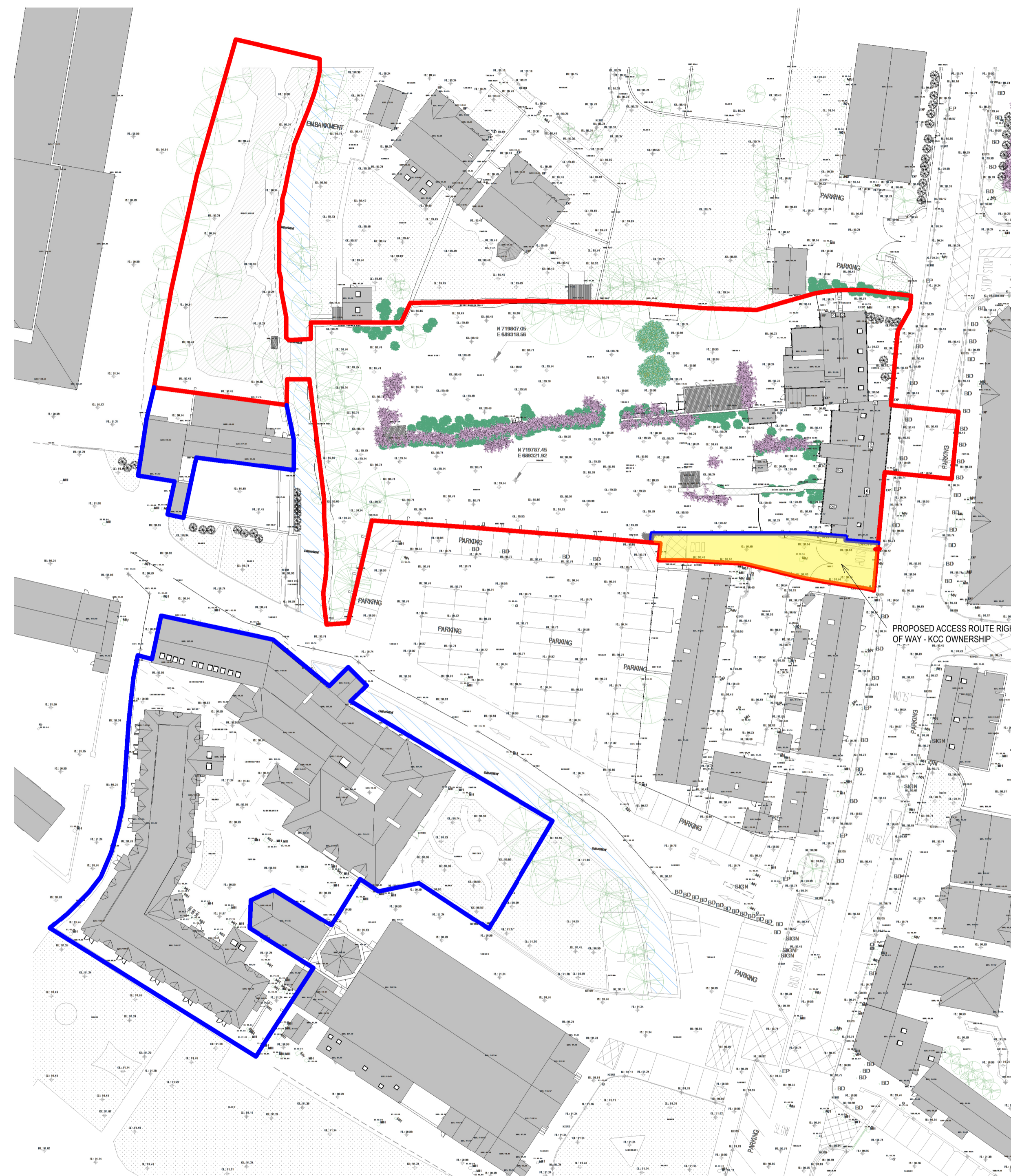
1 Existing Survey Site Plan Scale: 1:500
